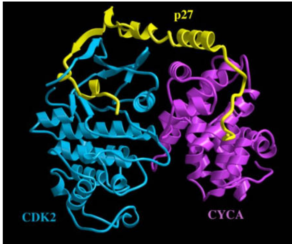
p27(Kip1)-CyclinA-Cdk2 Complex
