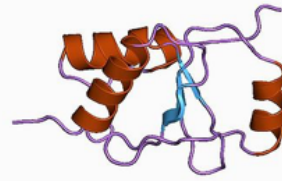
Kristallstruktur der BRCT-Domäne
